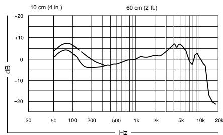
Tipica risposta in frequenza
