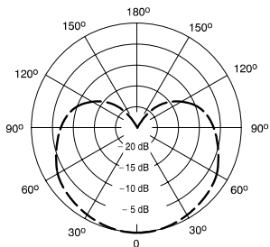
1000 Hz Richtcharakteristik
