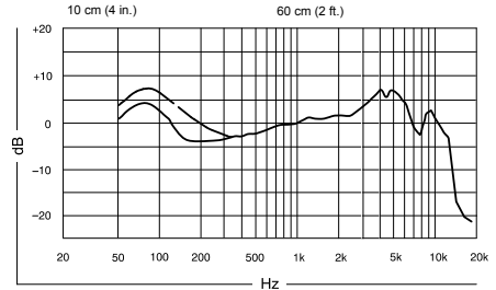
주파수 응답
