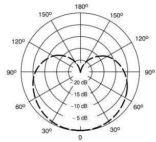
Diagramma polare tipico
