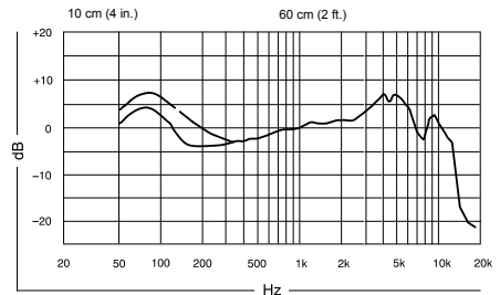
標準周波数特性
