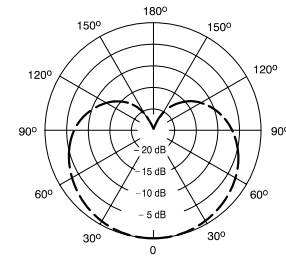
1000 Hz Типичная полярная диаграмма
