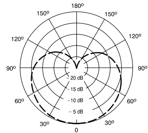
Courbe de directivité typique
