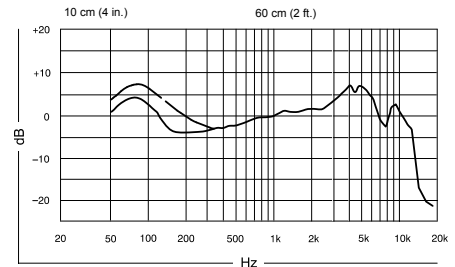
Типичная частотная характеристика
