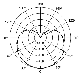
Padrão polar
