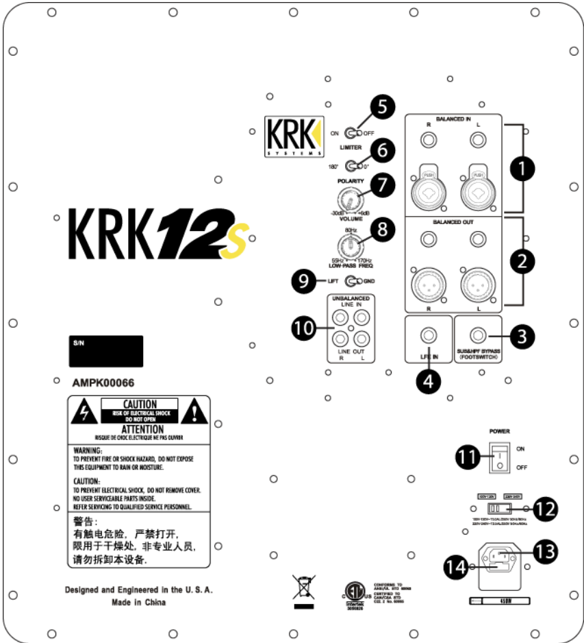
Figure 2.1 - Système de commande du panneau arrière
