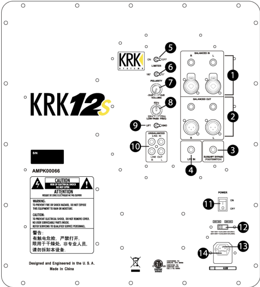
Figura 2.1 – Controles del Sistema en el Panel Trasero
