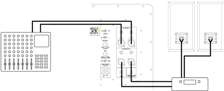
Figure 3.2 - Connexion du Subwoofer à des moniteurs de studio passifs
