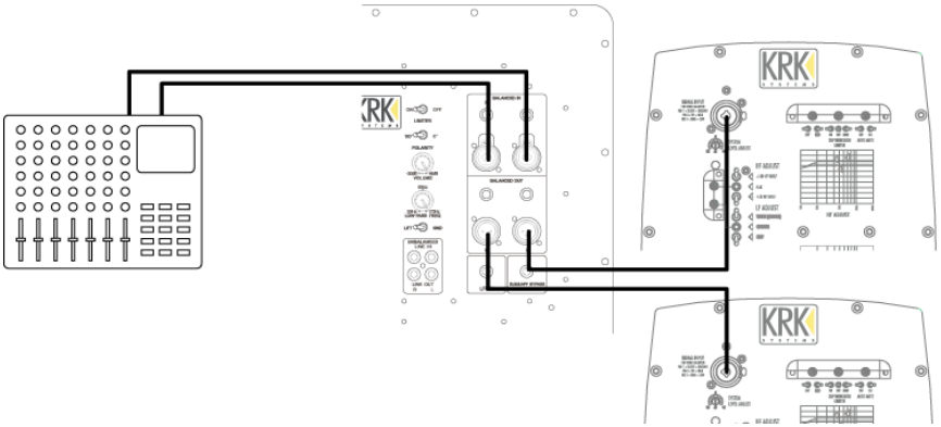
Figure 3.1 - Connexion du subwoofer à des moniteurs actifs
