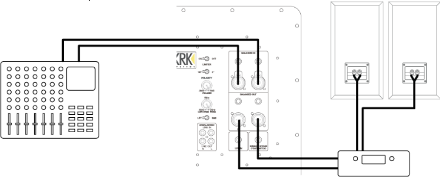
Figura 3.2 – Conexión del altavoz de bajos con Monitores Pasivos de Estudio
