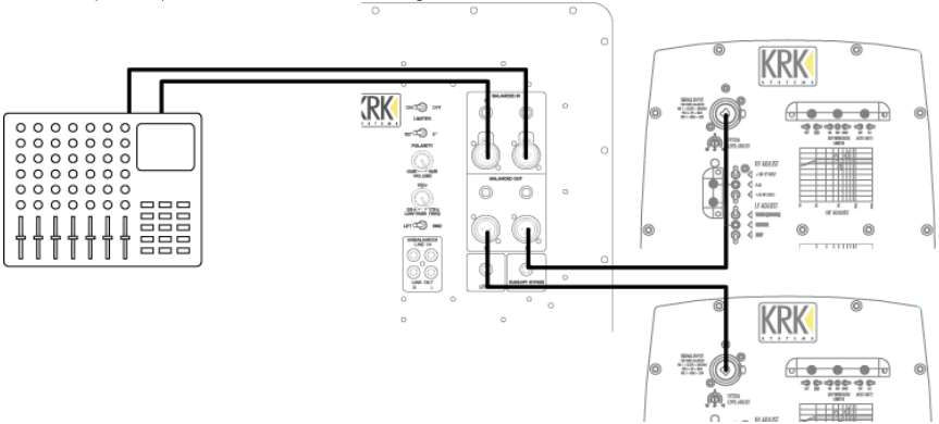
Figura 3.1 – Conexión del altavoz de bajos con Monitores Activos de Estudio
